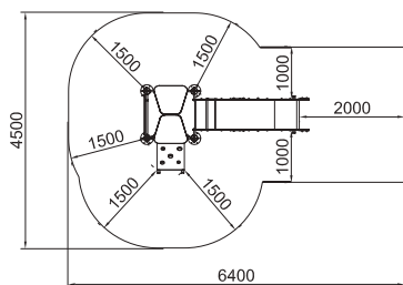
LD191.09.4 TORRE-TOBOGAN CASCABEL CON COLUMPIO
