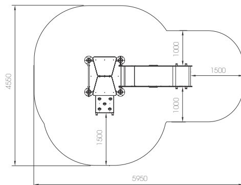
LD191.09.3 TORRE TOBOGAN ARBOL CON COLUMPIO
