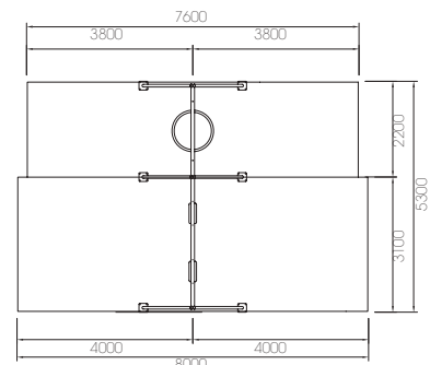
LD170.12.2 ESTRUCTURA COLUMPIO 3 ASIENTOS (2+1 CESTA)
