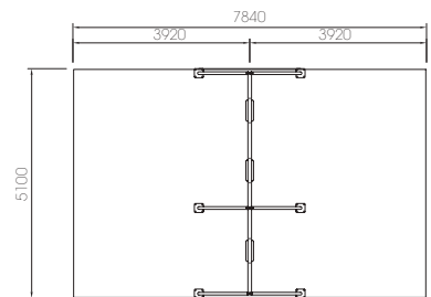
LD170.12.2 ESTRUCTURA COLUMPIO 3 ASIENTOS (2+1 CESTA)
