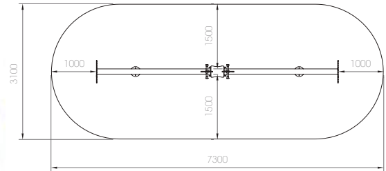
LD119.13 MODULAR MARINO ADAPTADO
