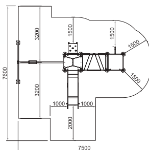
LD191.09.5 CONJUNTO 2 TORRES-CASCABEL CON COLUMPIO
