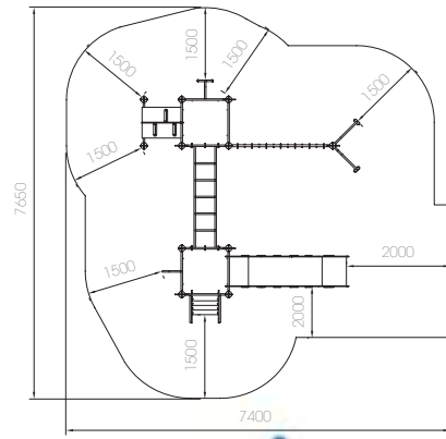
LD190.07.1 PUENTE MARINO
