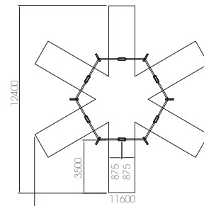
LD171.02 ESTRUCTURA HEXACOLUMPIO (6)
