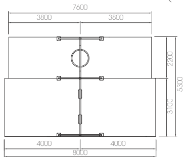
LD170.12.1 ESTRUCTURA COLUMPIO 3 ASIENTOS (2+1)
