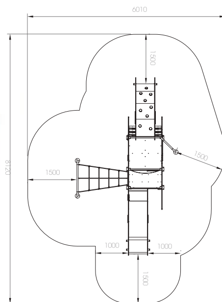
LD102.01 CANGREJO acceso escalera
