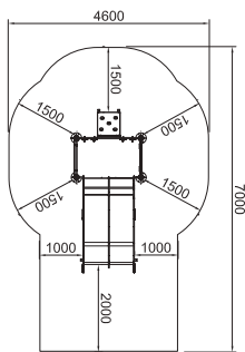
LD191.06.5 TORRE DOBLE TOBOGAN CASCABEL
