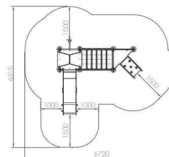
LD191.05.6 PUENTE COLGANTE CON ESCALERA
