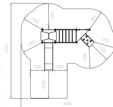
LD191.05.1 PUENTE MARINO TEJADO
