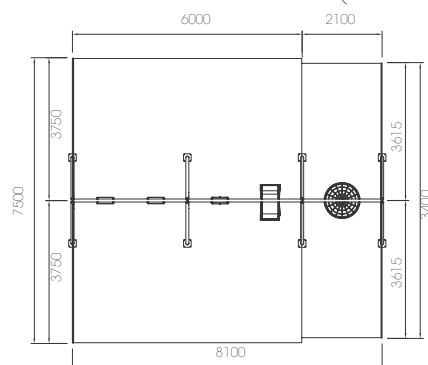
LD170.12.6 ESTRUCTURA COLUMPIO 5 ASIENTOS (2+2+1 CESTA)
