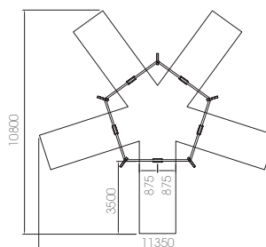
LD171.01 ESTRUCTURA PENTACOLUMPIO (5)
