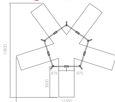
LD171.01 ESTRUCTURA PENTACOLUMPIO
