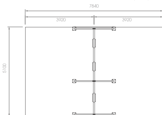
LD170.14 ESTRUCTURA COLUMPIO 4 ASIENTOS (1+2+1)
