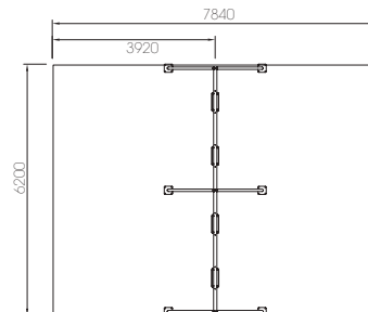
LD170.14.4 ESTRUCTURA COLUMPIO 4 ASIENTOS (2+2)
