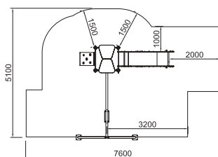
LD191.09.4 TORRE-TOBOGAN CASCABEL CON COLUMPIO
