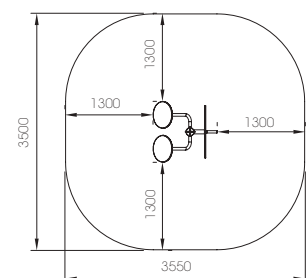
LD149.01 MAQUINA TIMON Y VOLANTE ADAPTADA
