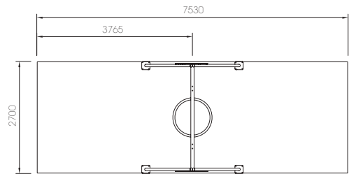
LD170.12.1 ESTRUCTURA COLUMPIO 3 ASIENTOS (2+1)
