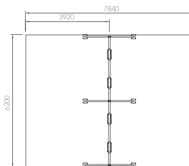
LD170.12.6 ESTRUCTURA COLUMPIO 5 ASIENTOS (2+2+1 CESTA)
