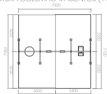
LD170.14.4 ESTRUCTURA COLUMPIO 4 ASIENTOS (2+2)
