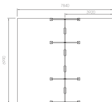
LD170.14 ESTRUCTURA COLUMPIO 4 ASIENTOS (1+2+1)
